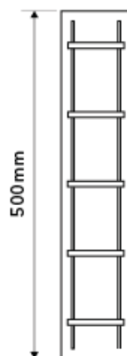
ELEVATION
